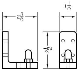
24 - KIT SIDELITE BOTTOM PIVOT
